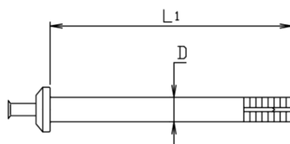
図1.1 アンカーの形状
